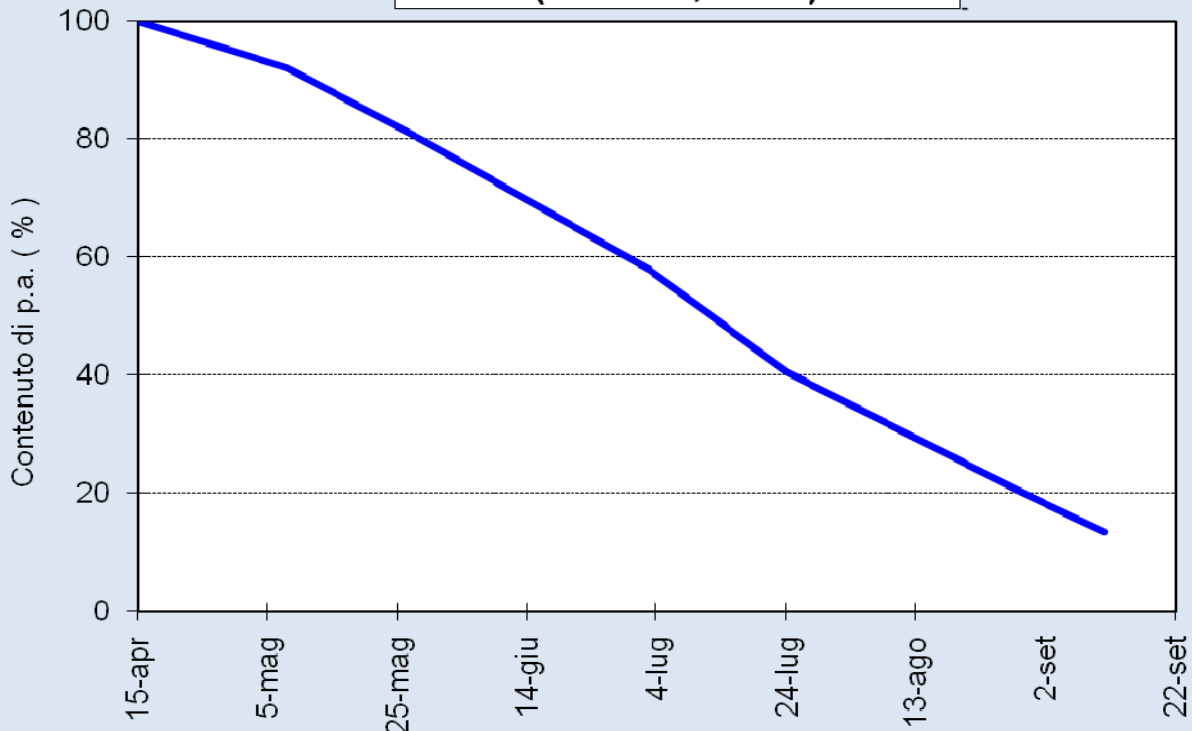
Curva di scarico di Isonet L (Cesena, 2006)
